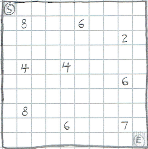
Nurikabe Path
